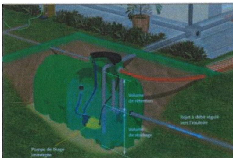
Cuve de stockage et rétention
